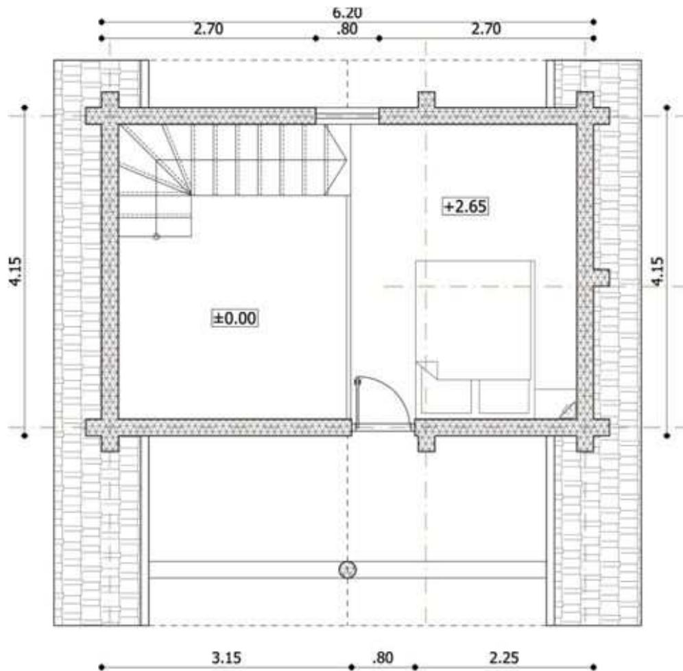
Plan etaj S=12.85 mp
